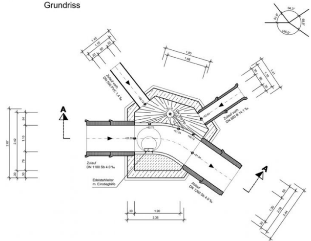
Schacht 0404355 Grundriss
