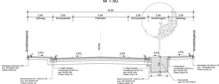
RQ 1 Stat. 0+080,00 M 1:50
