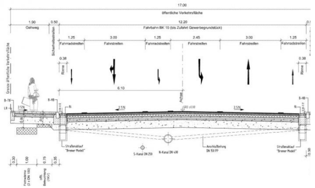
Ausbauquerschnitt A - A Einmündungsbereich Planstraße 1
