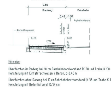
Ausbauquerschnitt III - III (Teilsanierung)
