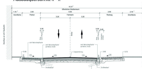
Ausbauquerschnitt II - II
